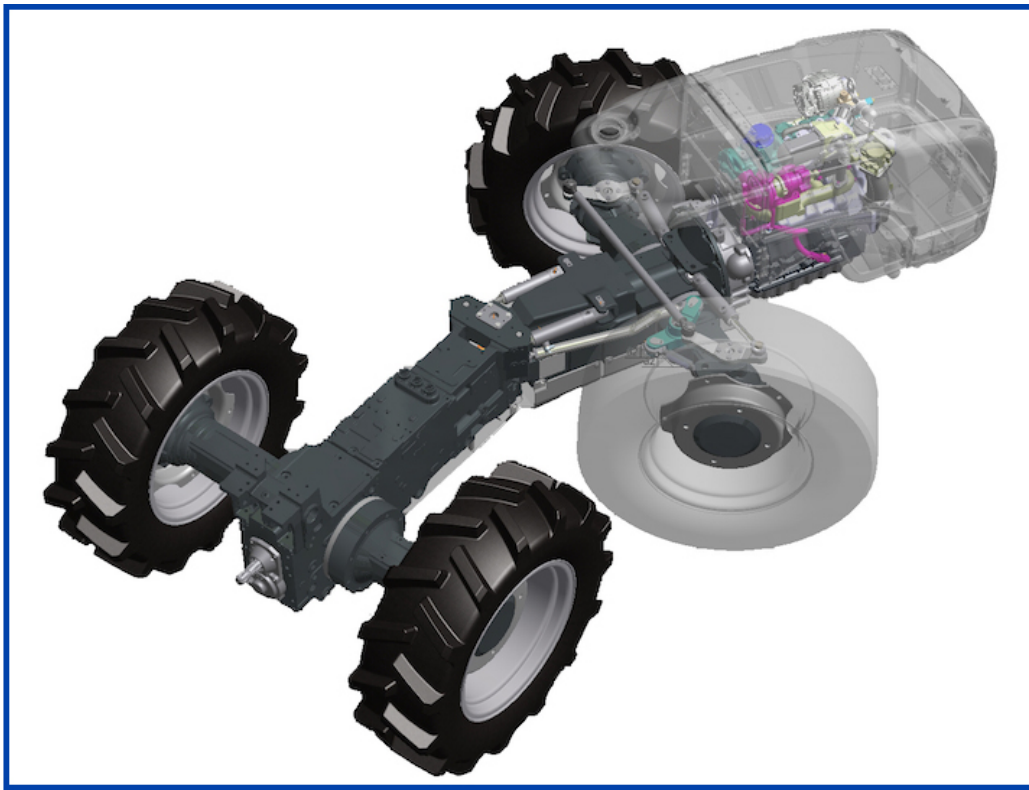
Sistema Dualsteer® di BCS
